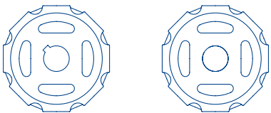
AVEC CLAVETTE SANS CLAVETTE
